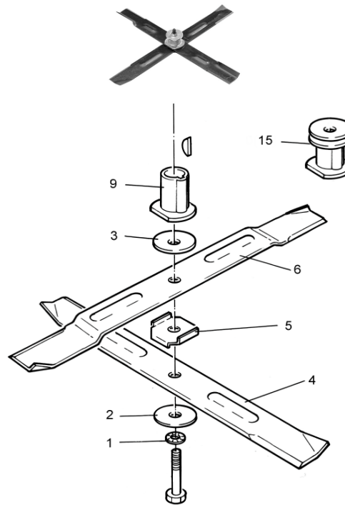
DOPPELMESSER SCHNEIDSYSTEM
