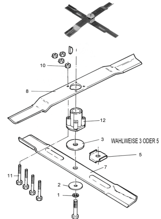
TAMDEMMESSER SCHNEIDSYSTEM
