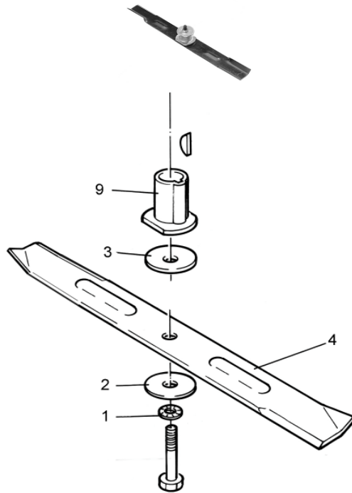
EINZELMESSER SCHNEIDSYSTEM
